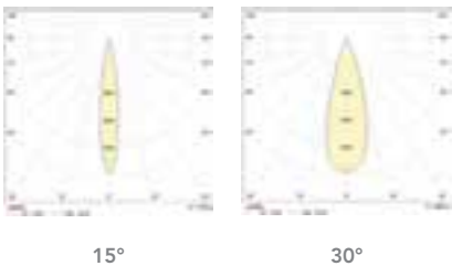
FOTOMETRÍAS
